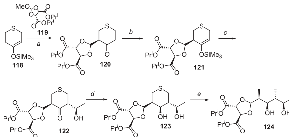
Scheme 14 a \text{ZnCl}_2 , \text{CH}_2\text{Cl}_2 , 55, 21 h, rt; b \text{LiHMDS} , THF, \text{TMSCl} , 1 h, -78^\circ\text{C} to >0^\circ\text{C} ; c \text{CH}_3\text{CHO} , \text{TiCl}_4 , \text{CH}_2\text{Cl}_2 , 5 min, -78^\circ\text{C} ; d \text{Et}_2\text{BOMe} , \text{NaBH}_4 , THF–MeOH, 1 h, -78^\circ\text{C} ; e Raney Ni, IPA, 24 h, 70^\circ\text{C} .
