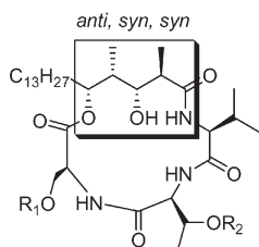
Stevastelin A: R_1 = \text{Ac} , R_2 = \text{SO}_3\text{H} Stevastelin B: R_1 = \text{Ac} , R_2 = \text{H}
