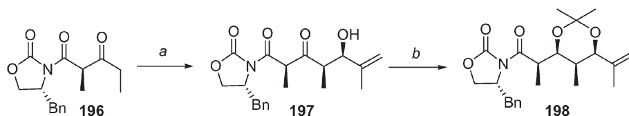
Scheme 25 a TiCl 4 , i -Pr 2 NEt, methacrolein, 0 °C, CH 2 Cl 2 ; b 1. Zn(BH 4 ) 2 , -78 °C, CH 2 Cl 2 ; 2. Me 2 C(OMe) 2 , CSA, 25 °C, CH 2 Cl 2 .
