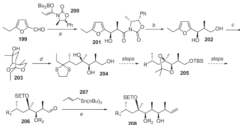
Scheme 26 a 200 , CH 2 Cl 2 , 199 ; b LiBH 4 , THF; c 1. Br 2 , MeCN, H 2 O; 2. Me 2 CuLi; 3. MeLi, CeCl 3 ; d TMSSCH 2 CH 2 STMS, TiCl 4 ; e 206 , 207 , BF 3 ·OEt, CH 2 Cl 2 .
